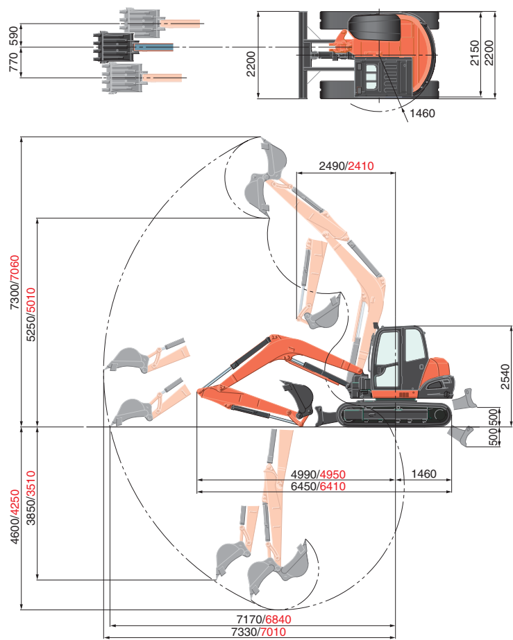
Balancier de 2100 mm Balancier de 1750 mm Unité:mm
